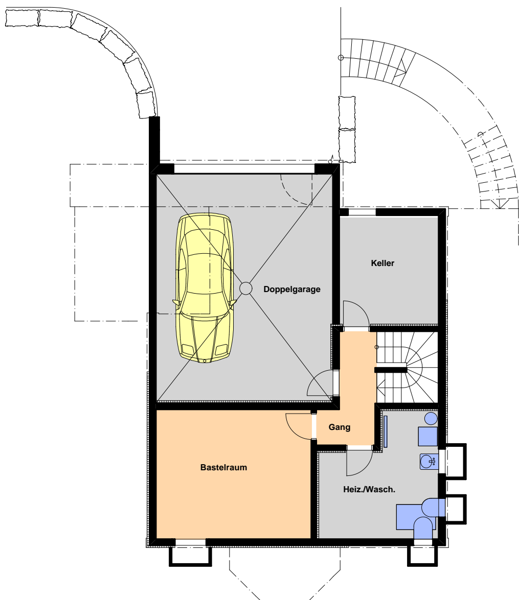
UNTERGESCHOSS
