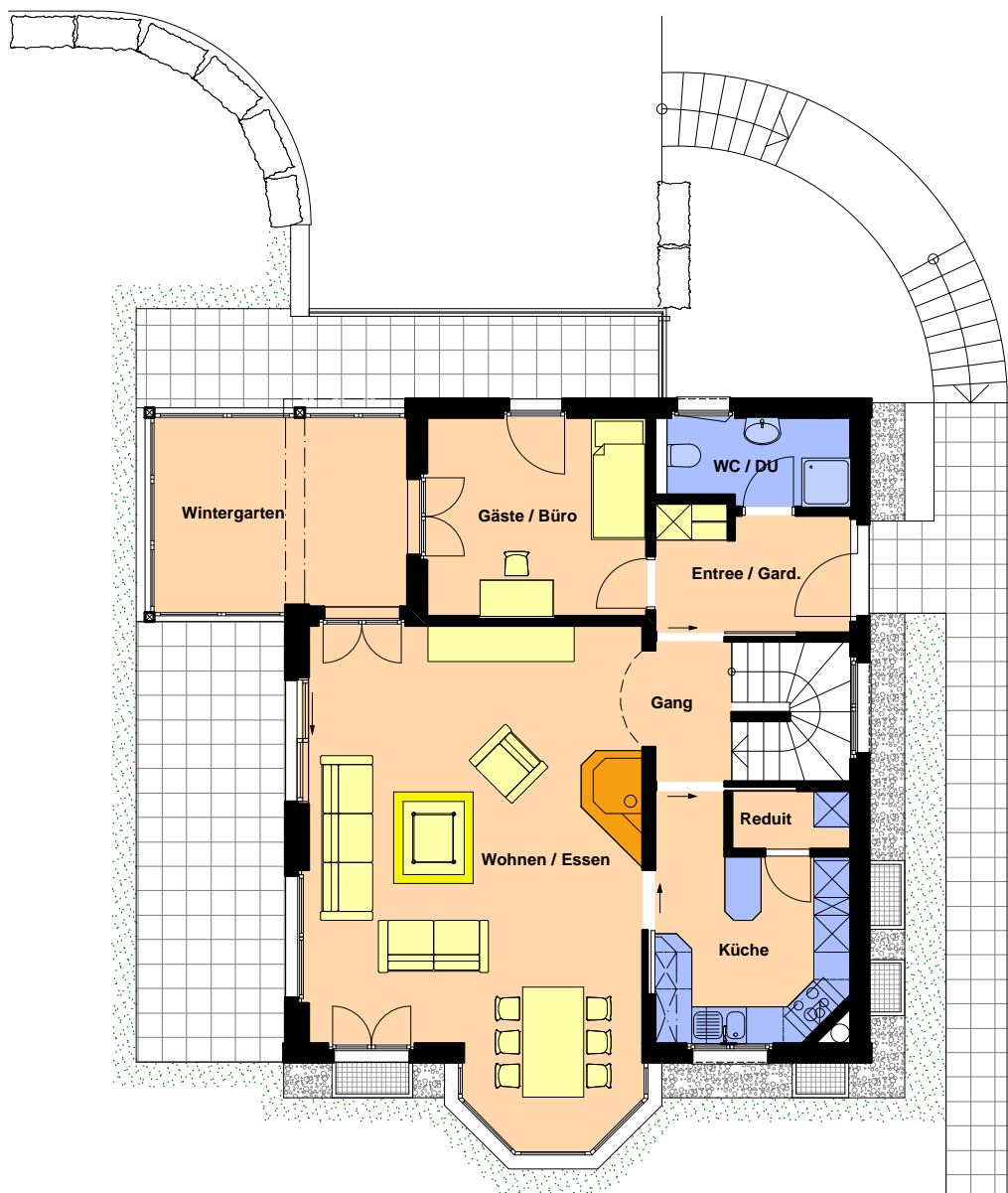
ERDGESCHOSS
